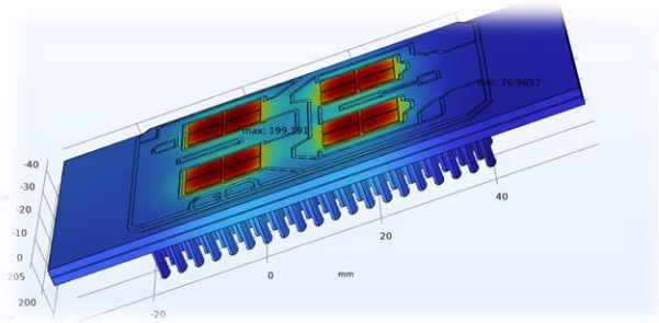
Fig. 10. Thermal simulation
